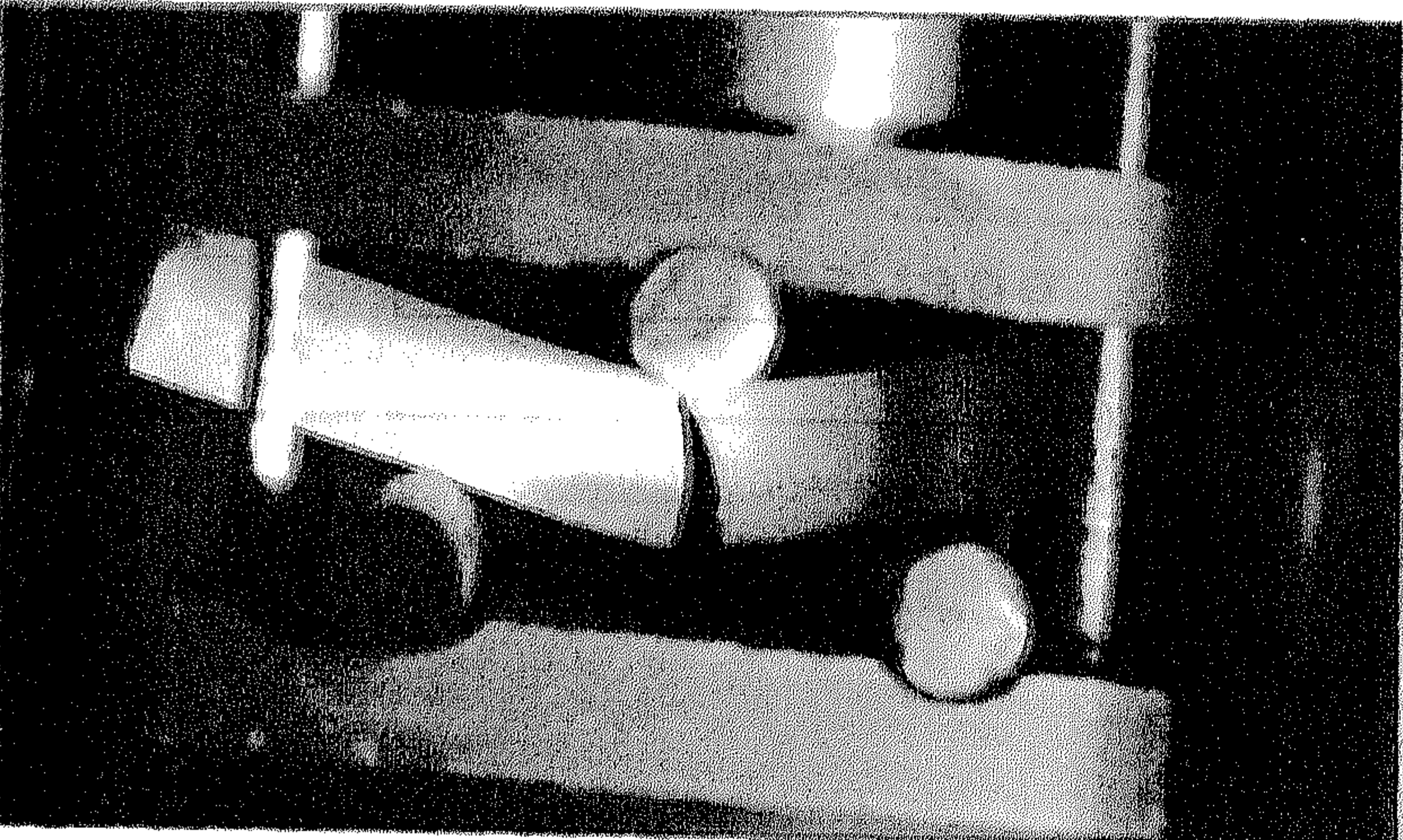
العينة (١٨) عند ضغط انحناء ٤١ كجم/سم ٢
